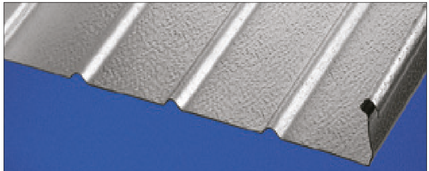
Arriba: Superficie gofrada. Abajo: Kalzip® AluPlusPatina.
